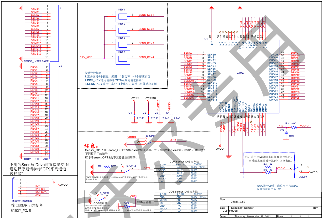
GT927 参考应用电路图
